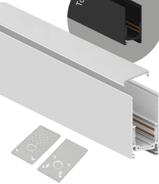
CABM1000 арт.41960 (1 м)/41962 (2 м) Шинопровод накладной Размеры, mm (1000/2000x26x53)
